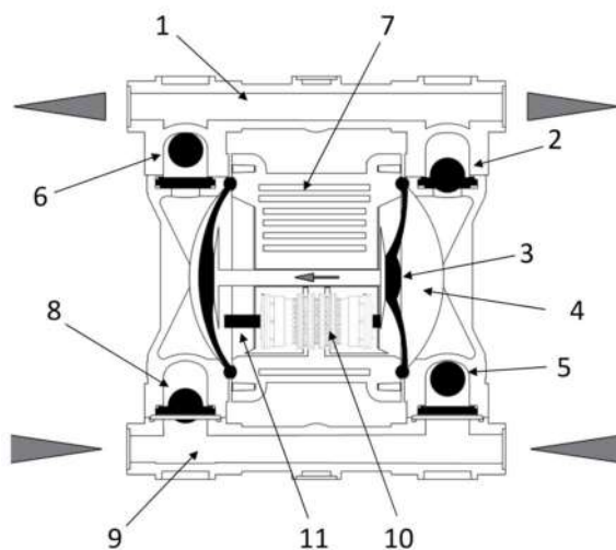
Рис. 2 : Конструкция насоса
